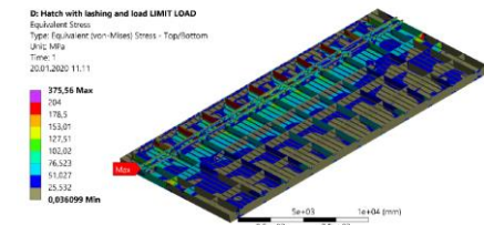
FEA
