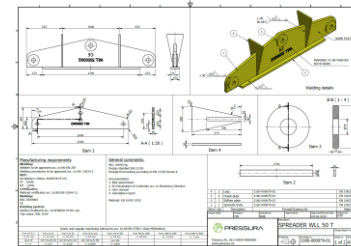
Teknisk tegning
